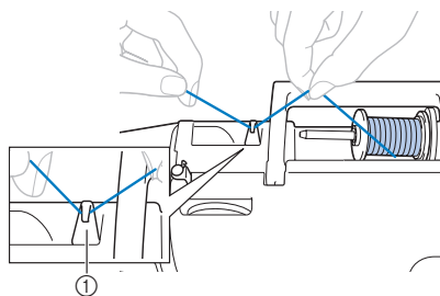
① Нитенаправитель
